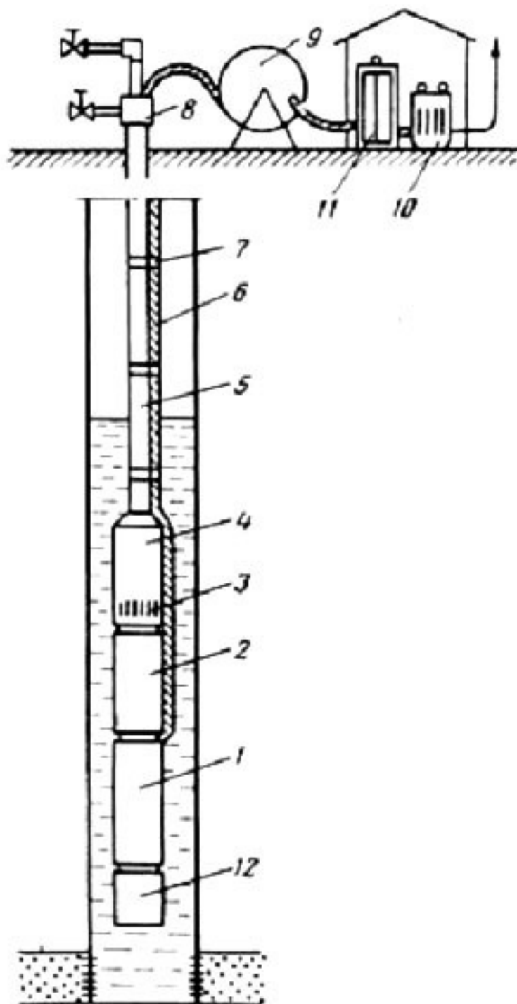
Рис. 10.1. Общая схема установки погружного центробежного насоса:
