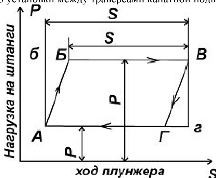
Рис. 11.3. Теоретическая динамограмма ШСН
