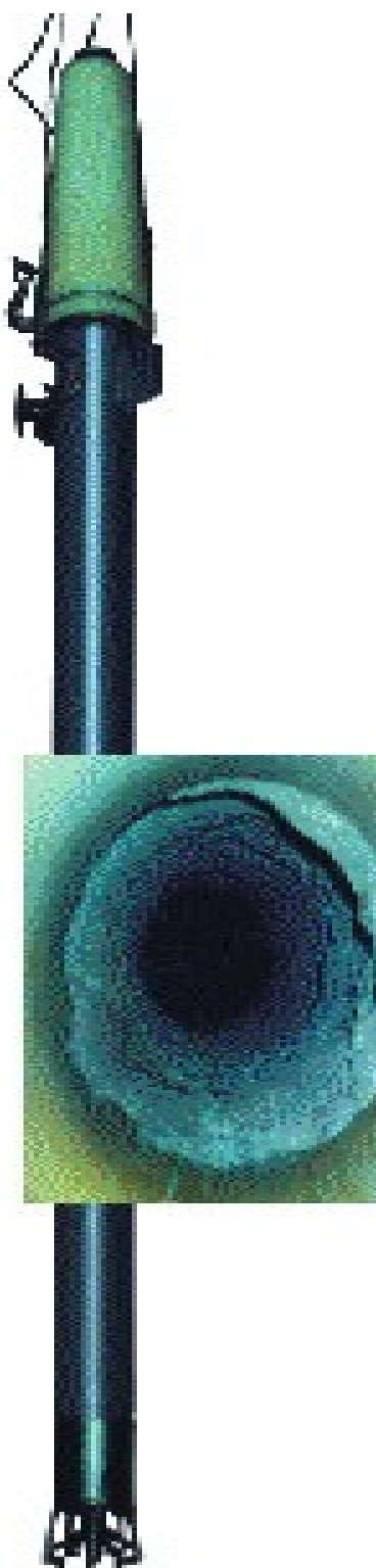
Рис. 4.29. Общий вид бурового снаряда: 1 – буровой наконечник диаметром 270 мм; 2 – буровые трубы диаметром 200 мм; 3 – высоковольтный ввод
