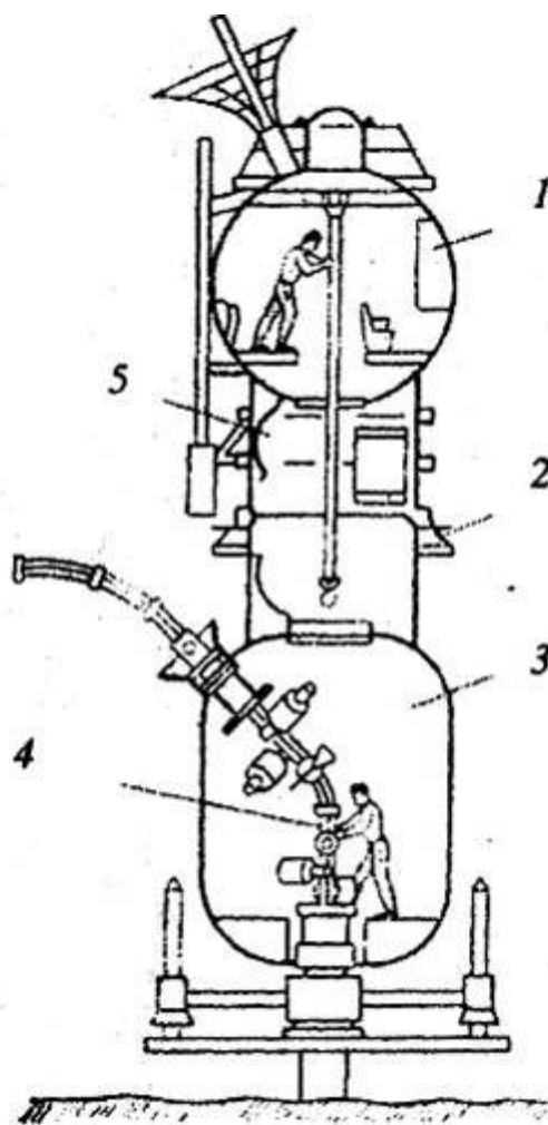
Рис. 17.4. Схема “сухого” заканчивания морской скважины
