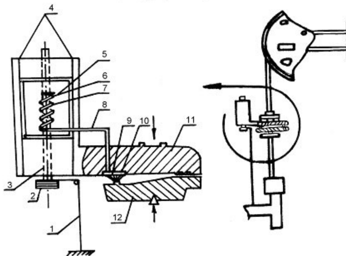
Рис. 11.2. Принципиальная схема гидравлического динамографа и его установки между траверсами канатной подвески:
