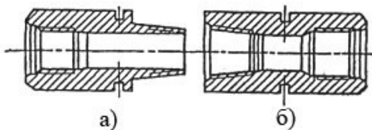
Рис. 4.21. Бурильный замок: а – замковый ниппель; б – замковая муфта
