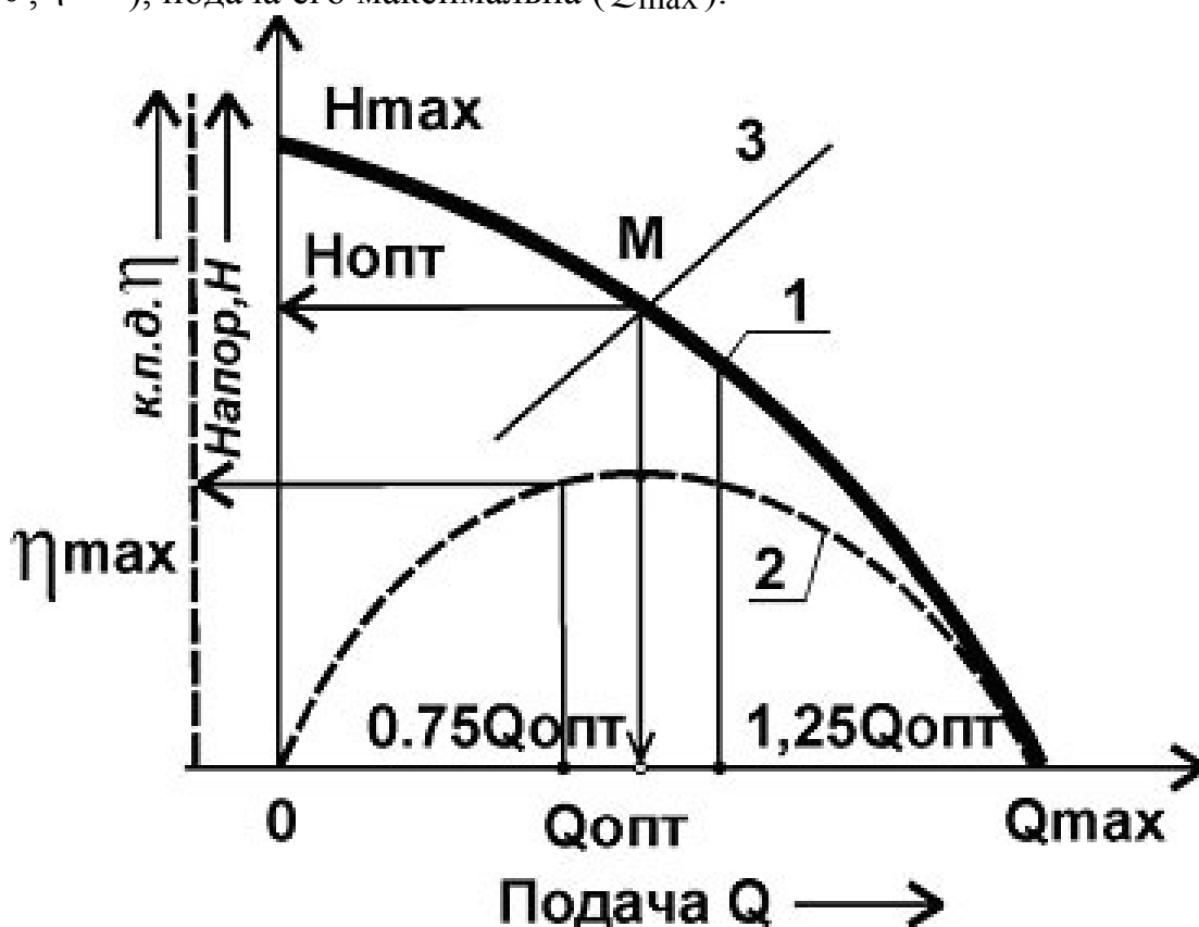
Рис. 10.2. Гидравлическая характеристика ПЭЦН
