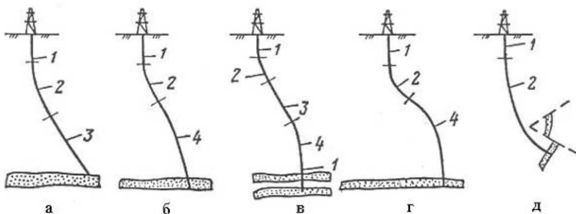
Рис. 4.27. Типы профилей наклонно-направленных скважин:
