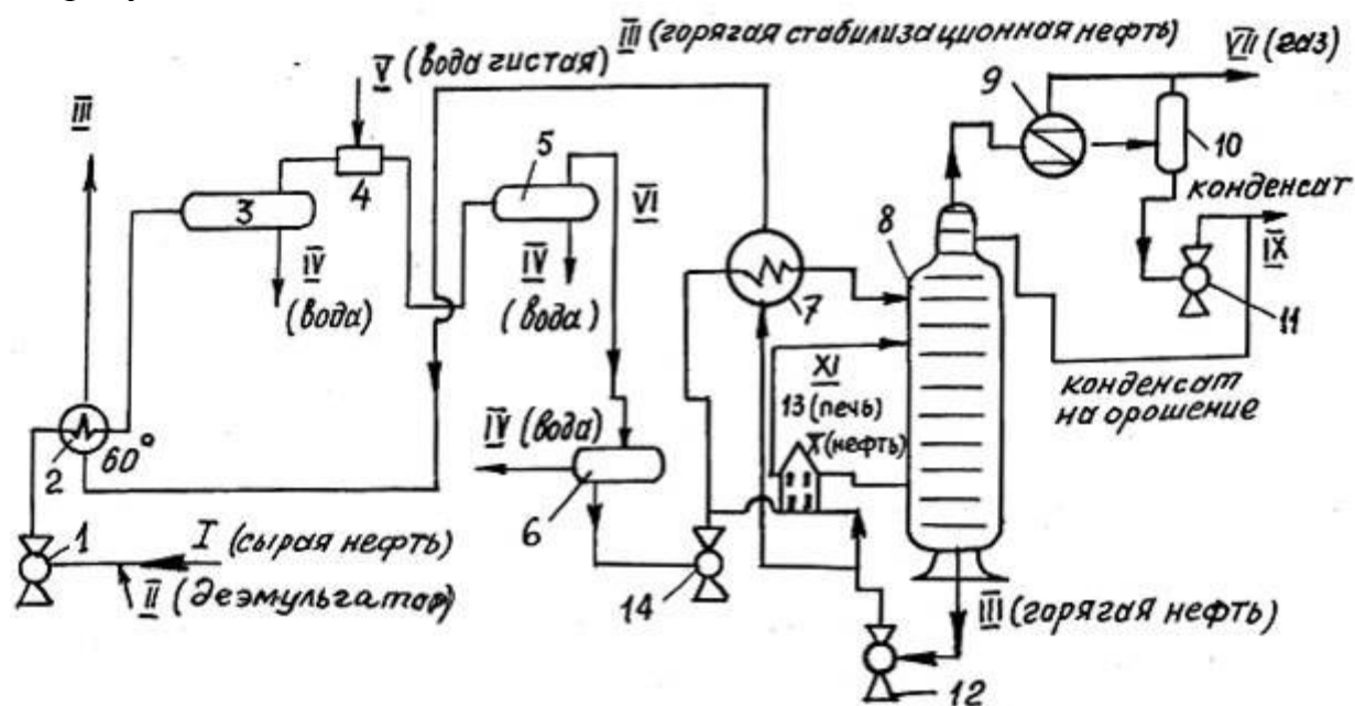
Рис. 12.2. Технологическая схема УКПН:
