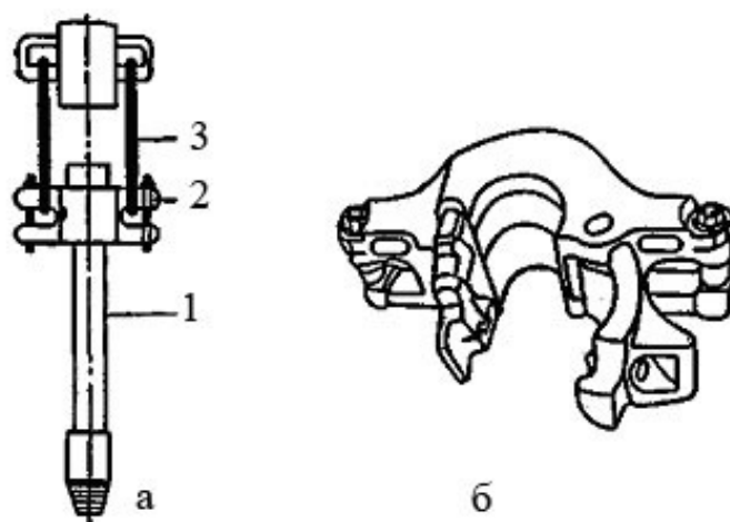
Рис. 4.14. Схема подвешивания бурильной трубы при спуско-подъемных операциях: а – схема; б – элеватор 1 – бурильная труба; 2 – элеватор; 3 – штроп
