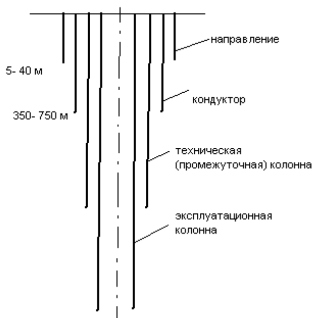
Рис. 4.5. Конструкция скважины
