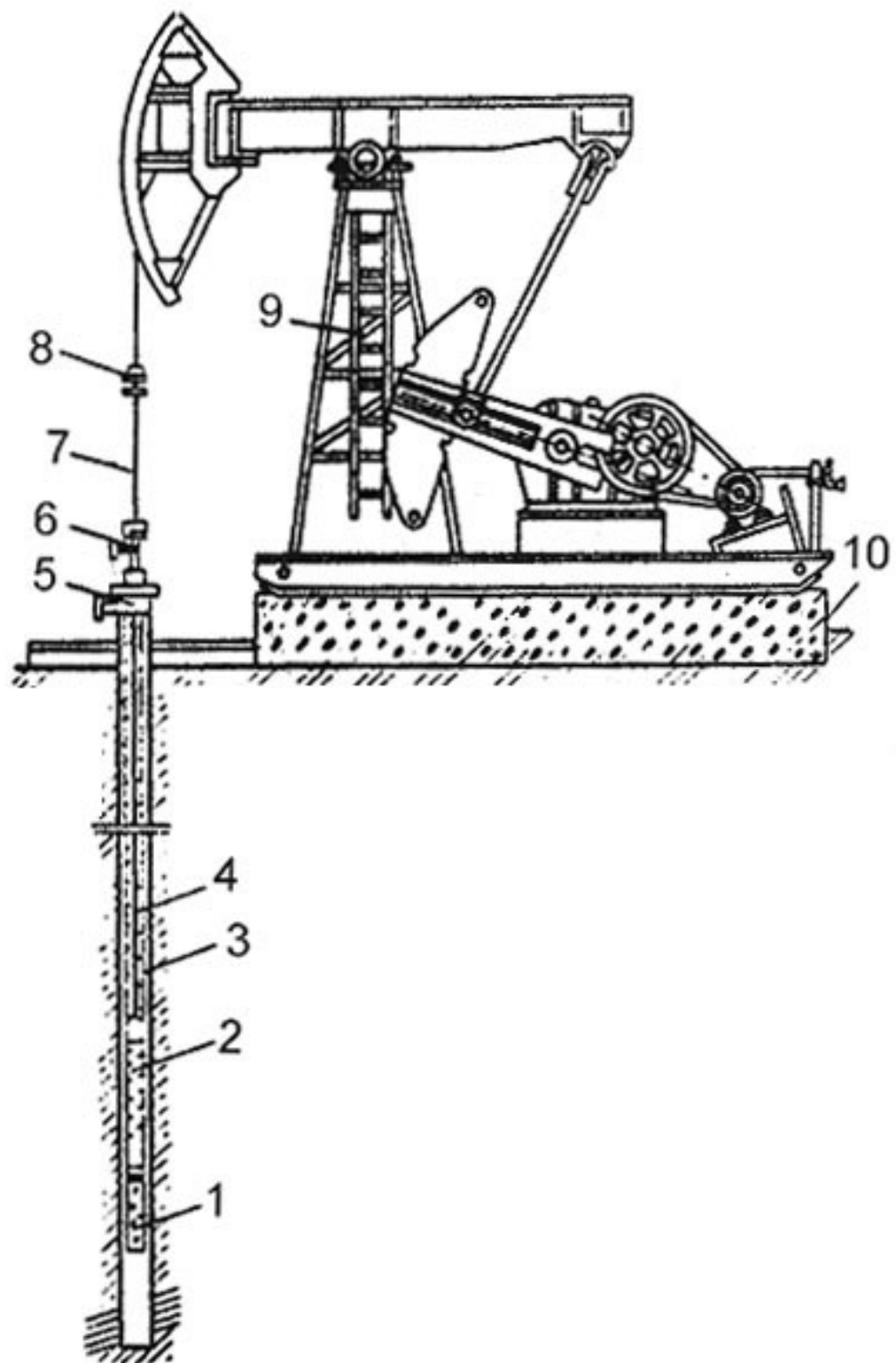
Рис. 9.1. Схема установки штангового скважинного насоса
