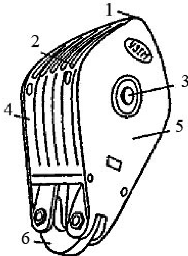
Рис. 4.13. Талевый блок: 1 – траверса; 2 – шкивы; 3 – ось; 4 – предохранительные кожухи; 5 – щеки; 6 – серьга
