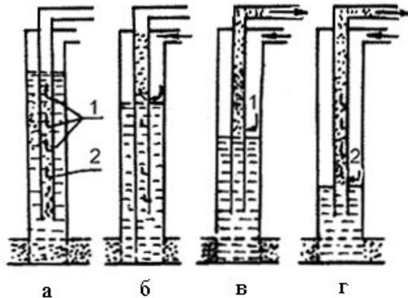
Рис. 8.1. Подъемники кольцевой системы: а – двухрядный; б – полуторорядный; в – однорядный
