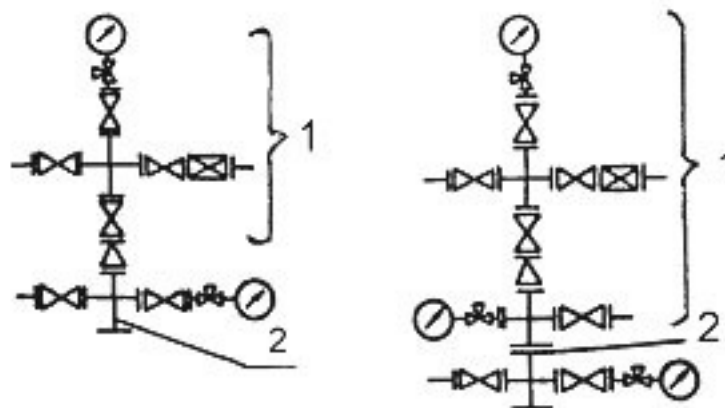
Рис. 7.5. Типовые схемы фонтанной арматуры: 1 – фонтанная елка; 2 – трубная обвязка
