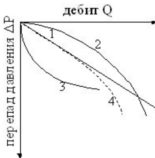
Рис. 7.7. Индикаторные диаграммы
