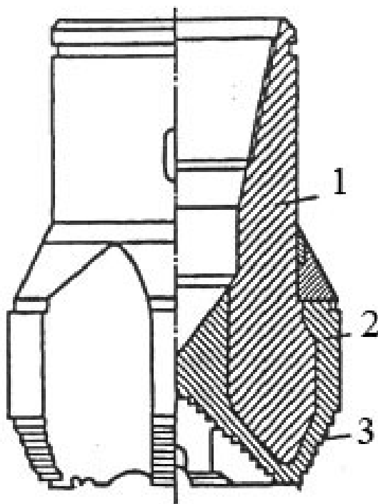
Рис. 4.20. Алмазное долото: 1 – корпус; 2 – матрица; 3 – алмазные зерна
