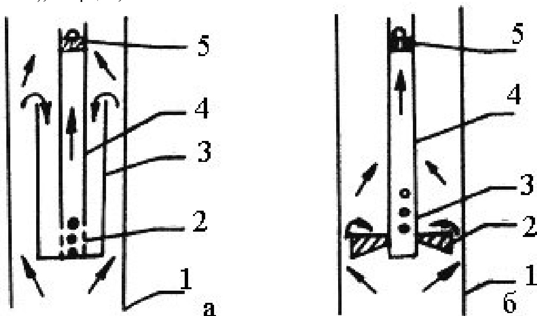
Рис. 11.5. Принципиальные схемы газовых якорей однокорпусного (а), однотарельчатого (б):
