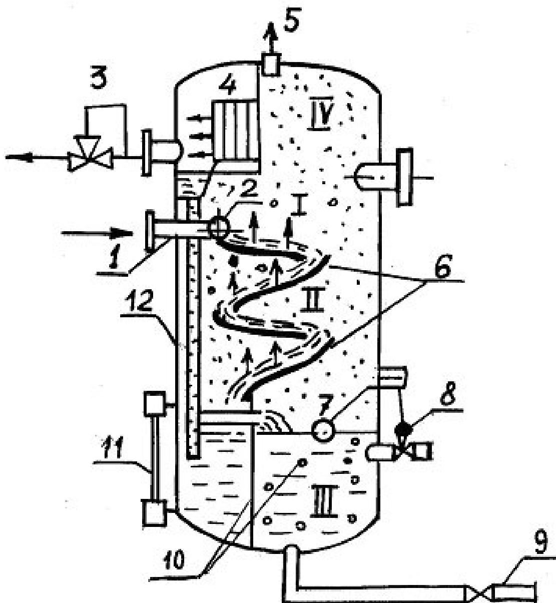
Рис. 12.3. Вертикальный сепаратор:
