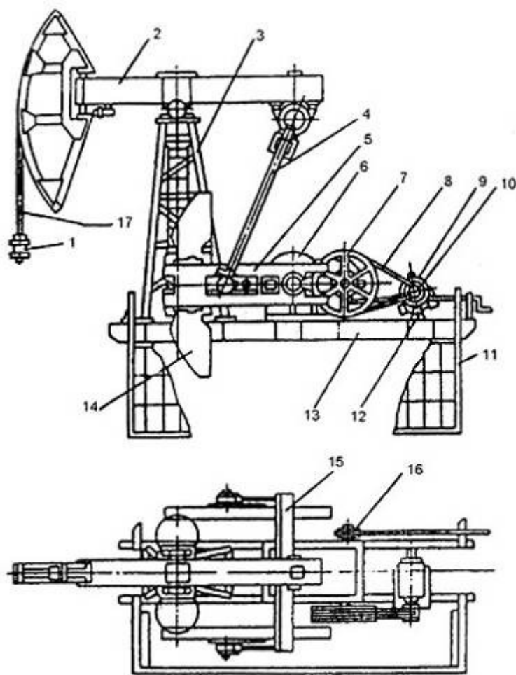
Рис. 9.4. Станок-качалка типа СКД:
