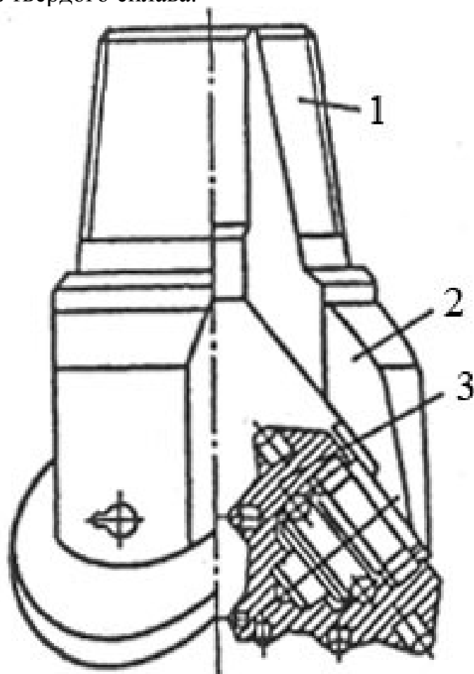
Рис. 4.19. Шарошечное долото: 1 – корпус с резьбовой головкой; 2 – лапа с опорой; 3 – шарошка
