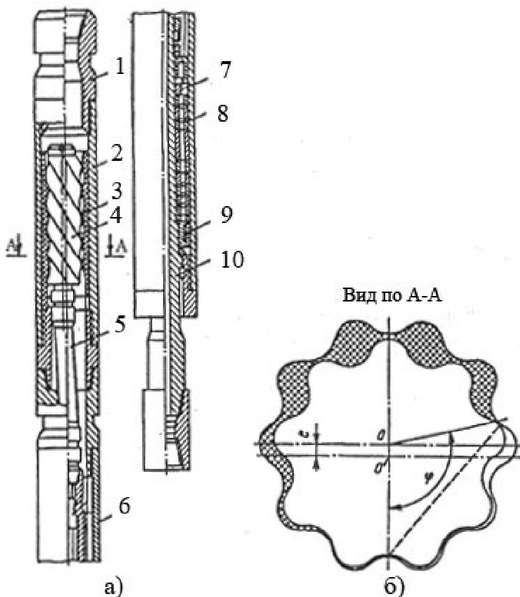
Рис. 4.17. Винтовой двигатель:
