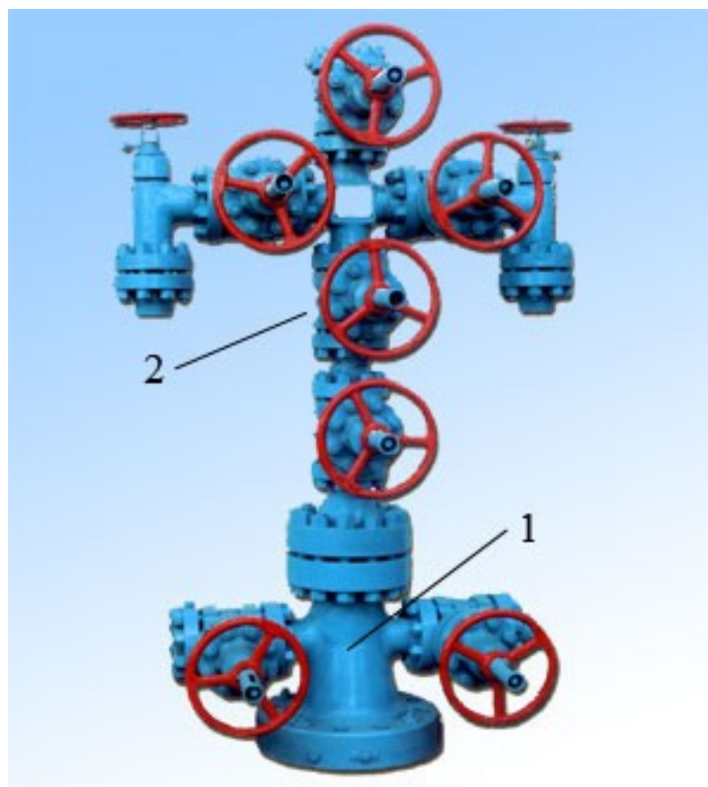
Рис. 7.2. Фонтанная арматура: 1 – трубная обвязка ; 2 – фонтанная елка
