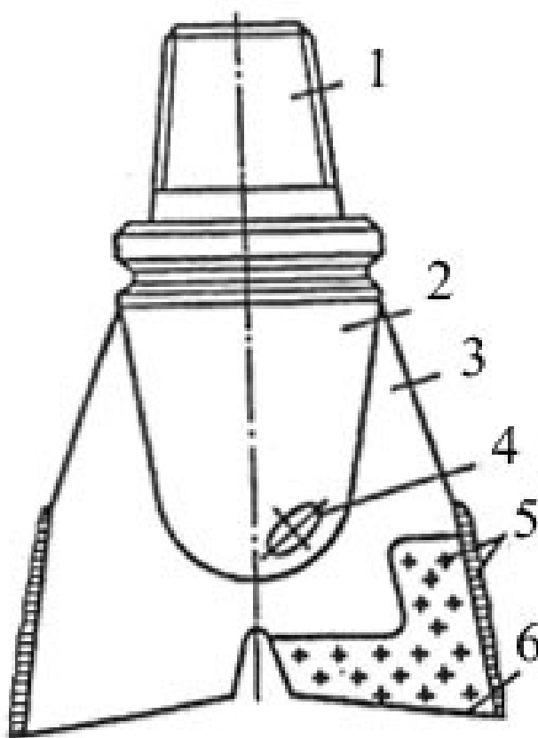
Рис. 4.18. Лопастное долото:
