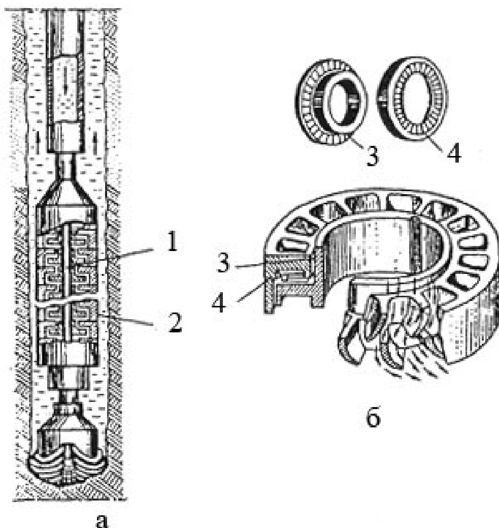
Рис. 4.16. Турбобур: а – общий вид; б – ступень турбобура; 1 – вал; 2 – корпус; 3 – ротор; 4 – статор
