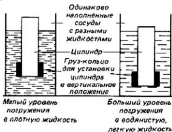
Рис. 2.2. Ареометр
