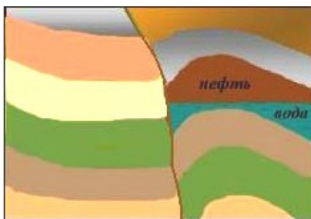
Рис. 3.3. Тектонически экранированная ловушка
