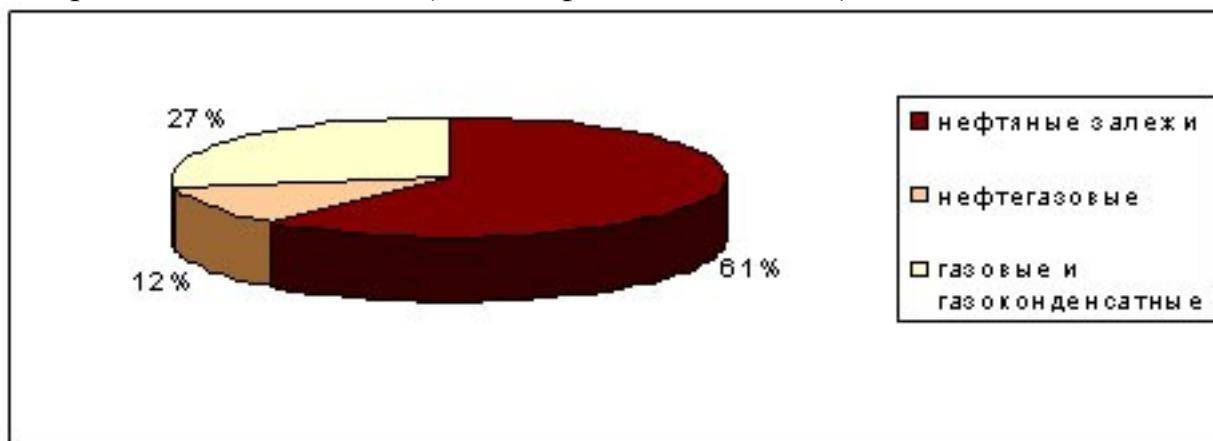
Рис. 3.10. Распределение залежей по типам углеводородов
