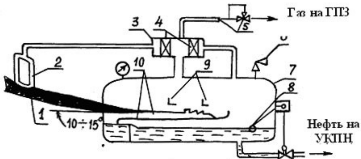
Рис. 12.4. Горизонтальный сепаратор с предварительным отбором газа:
