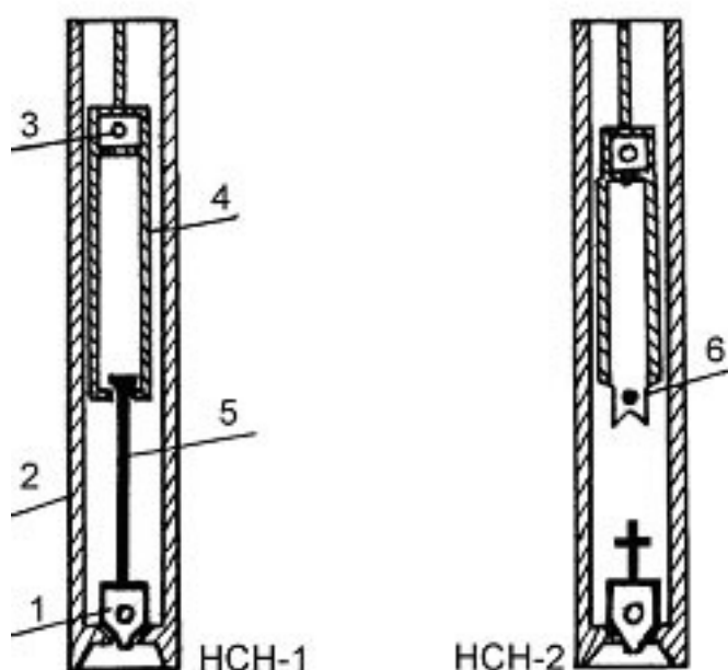
Рис. 9.3. Невставные скважинные насосы:
