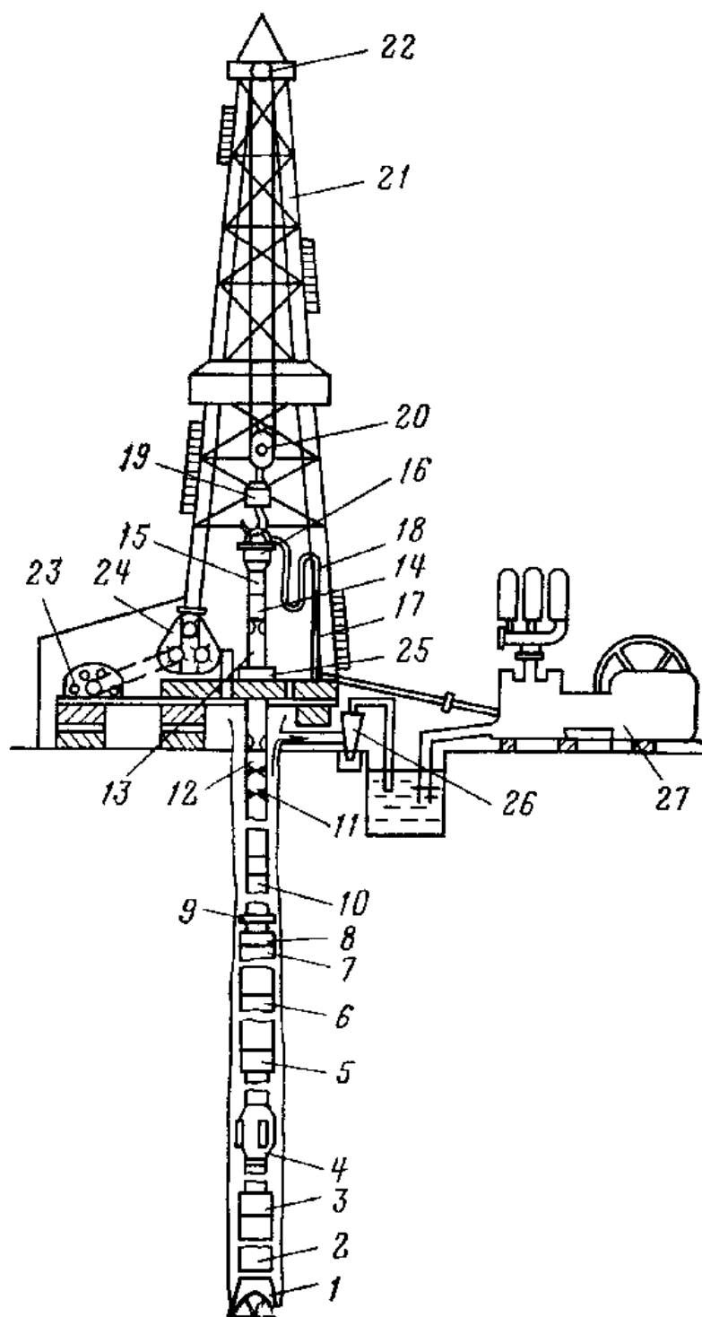
Рис. 4.9. Буровая установка:
