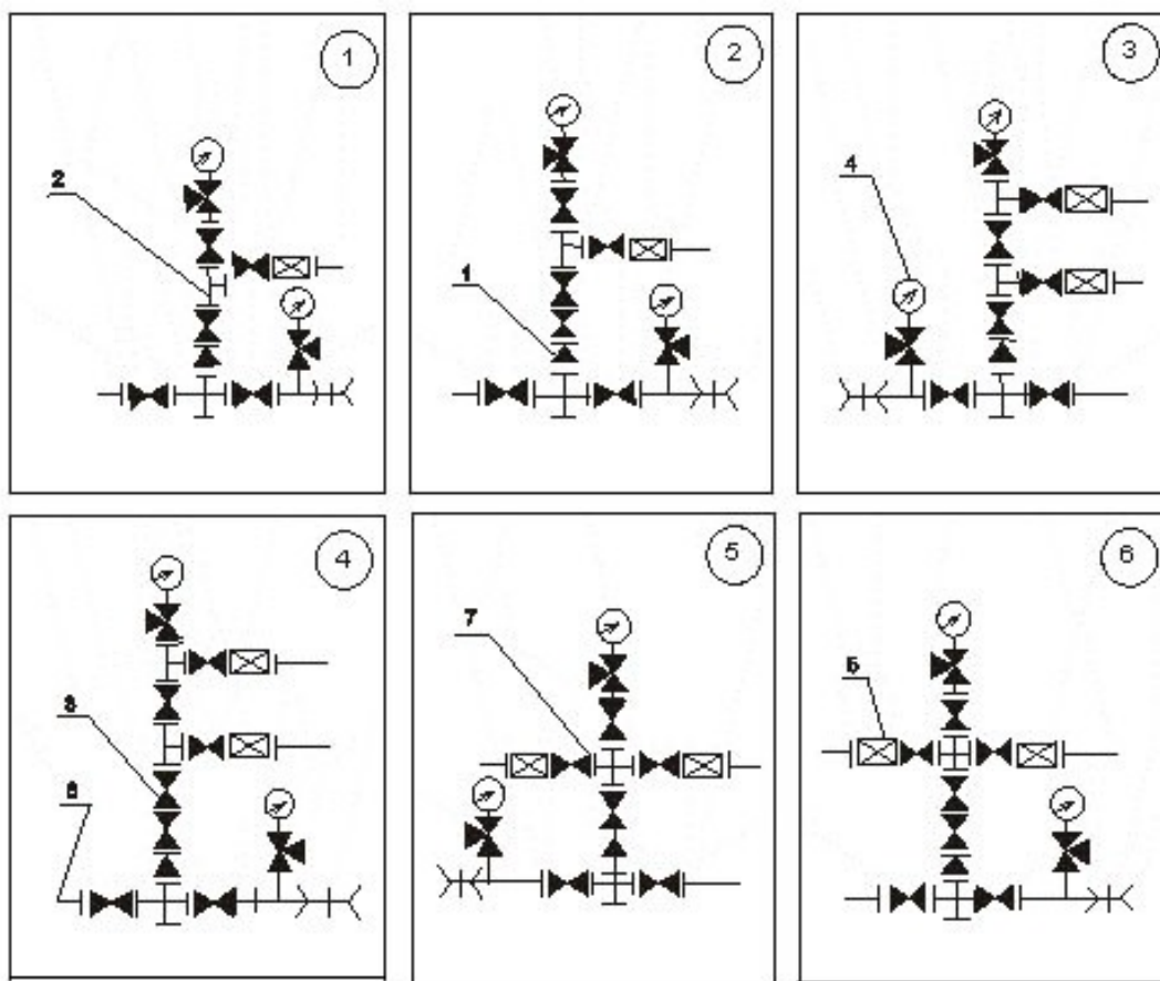
Рис. 7.4. Типовые схемы фонтанных елок:
