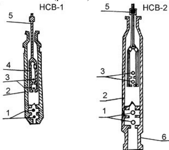
Рис. 9.2. Насосы скважинные вставные:
