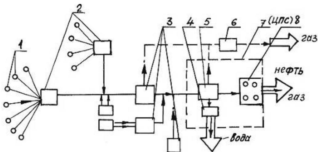
Рис. 12.1. Схема сбора и подготовки продукции скважин на нефтяном промысле:
