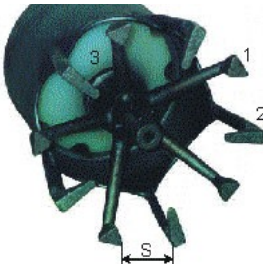
Рис. 4.30. Буровой наконечник диаметром 270 мм: 1 – высоковольтный электрод; 2 – заземленный электрод; 3 – изолятор бурового наконечника; S – расстояние между электродами
