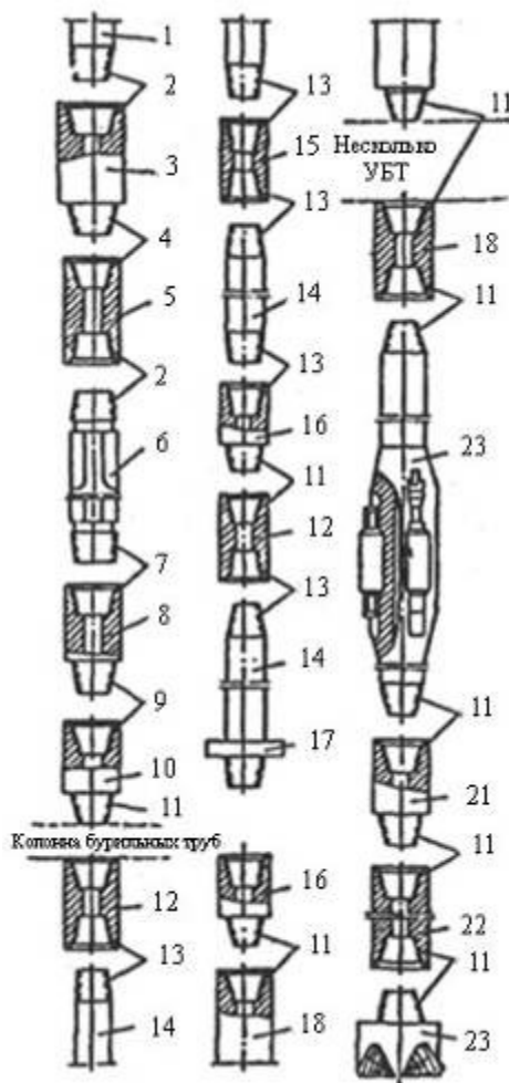
Рис. 4.24. Компоновка бурильной колонны:
