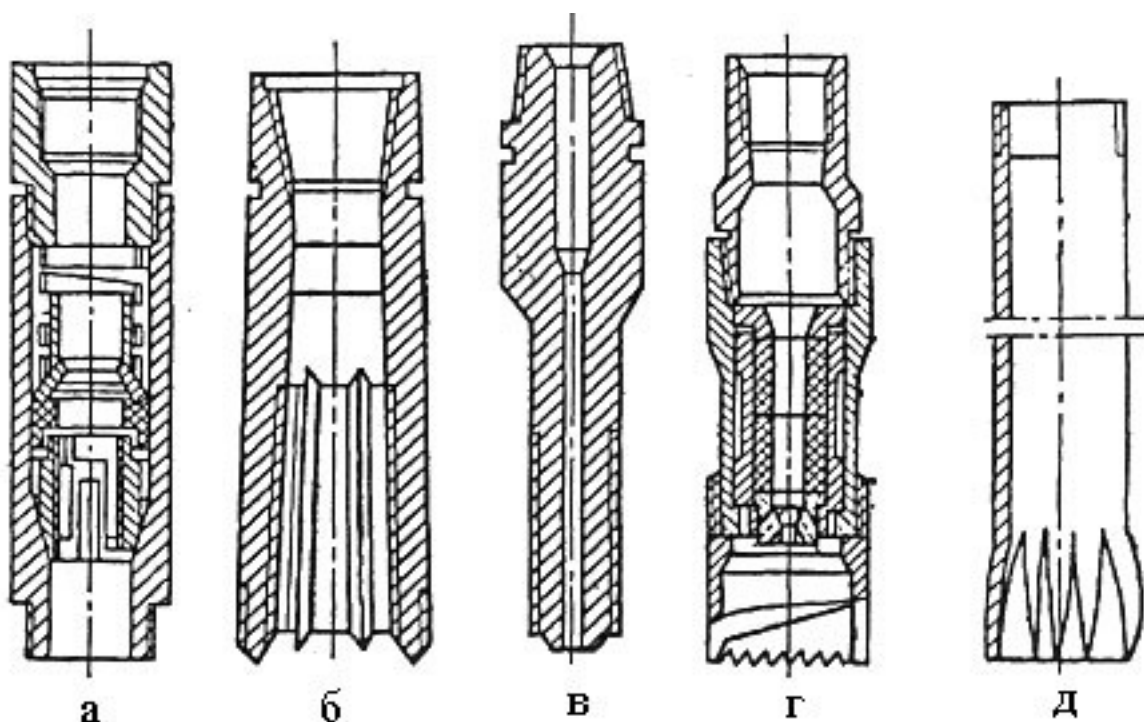
Рис. 4.26. Ловильные инструменты:
