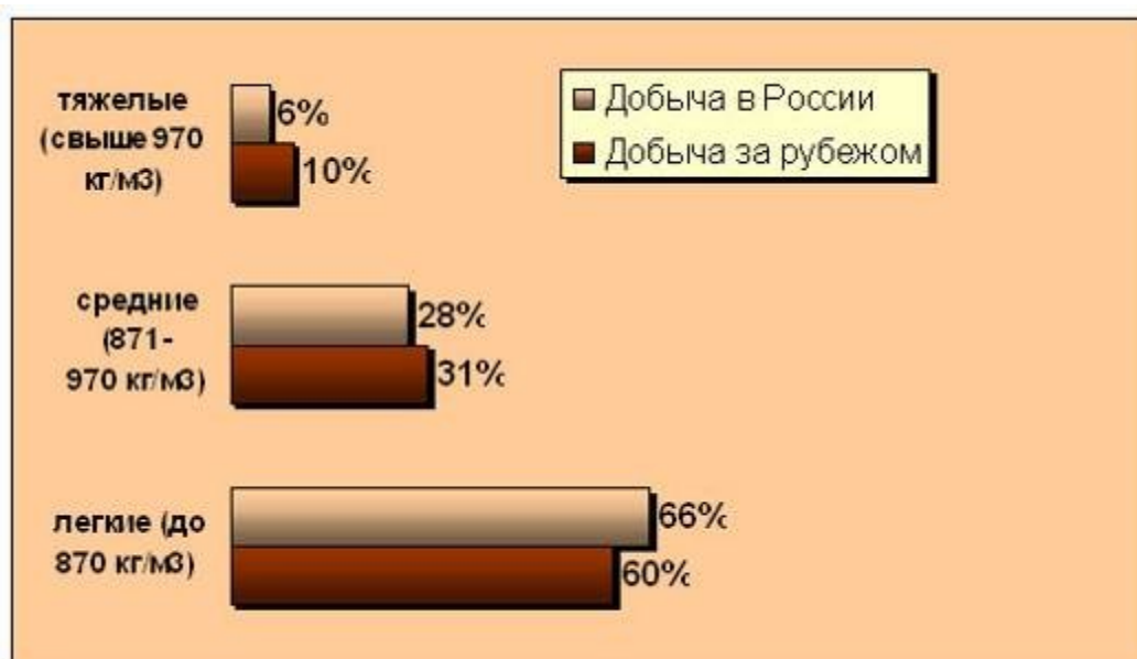
Рис. 2.3. Классификация нефти по плотности
