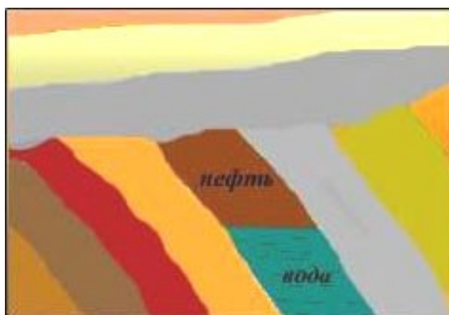
Рис. 3.4. Стратиграфически экранированная ловушка
