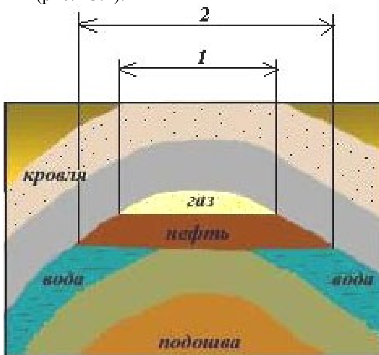
Рис. 3.1. Сводовая ловушка: 1 – внешний контур газоносности; 2 – внешний контур нефтеносности
