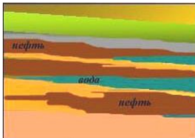
Рис. 3.2. Литологически экранированная ловушка
