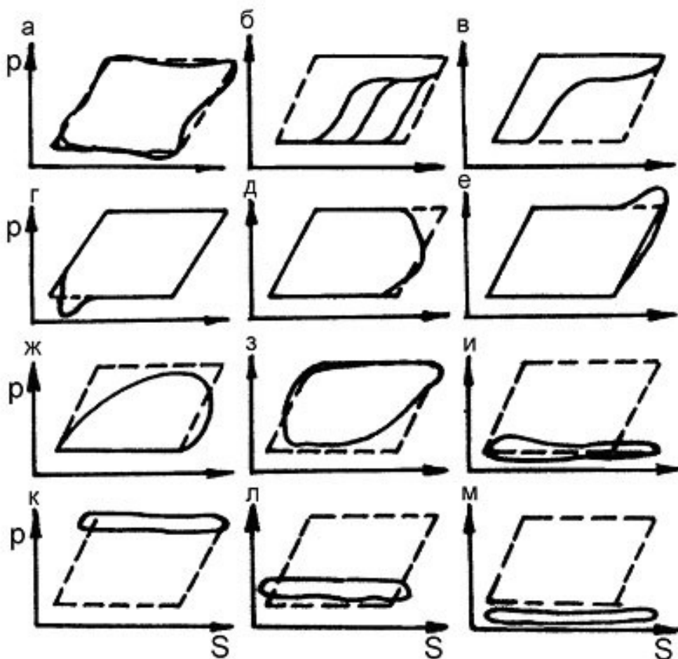
Рис. 11.4. Практические динамограммы работы ШСН: а – нормальная тихоходная работа; б – влияние газа; в – превышение подачи насоса над притоком в скважину; г – низкая посадка плунжера; д – выход плунжера из цилиндра невставного насоса; е – удары плунжера о верхнюю ограничительную гайку вставного насоса; ж – утечки в нагнетательной части; и – полный выход из строя нагнетательной части; к – полный выход из строя всасывающей части; л – полуфонтанный характер работы насоса; м – обрыв штанг (пунктиром показаны линии теоретической динамограммы); з – утечки во всасывающей части
