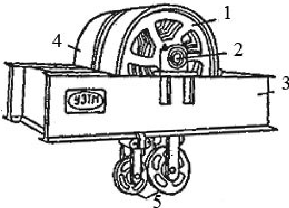
Рис. 4.12. Кронблок:
