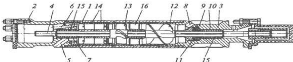
Рисунок 2 - Газосепаратор типа МН-ГСЛ [4]
