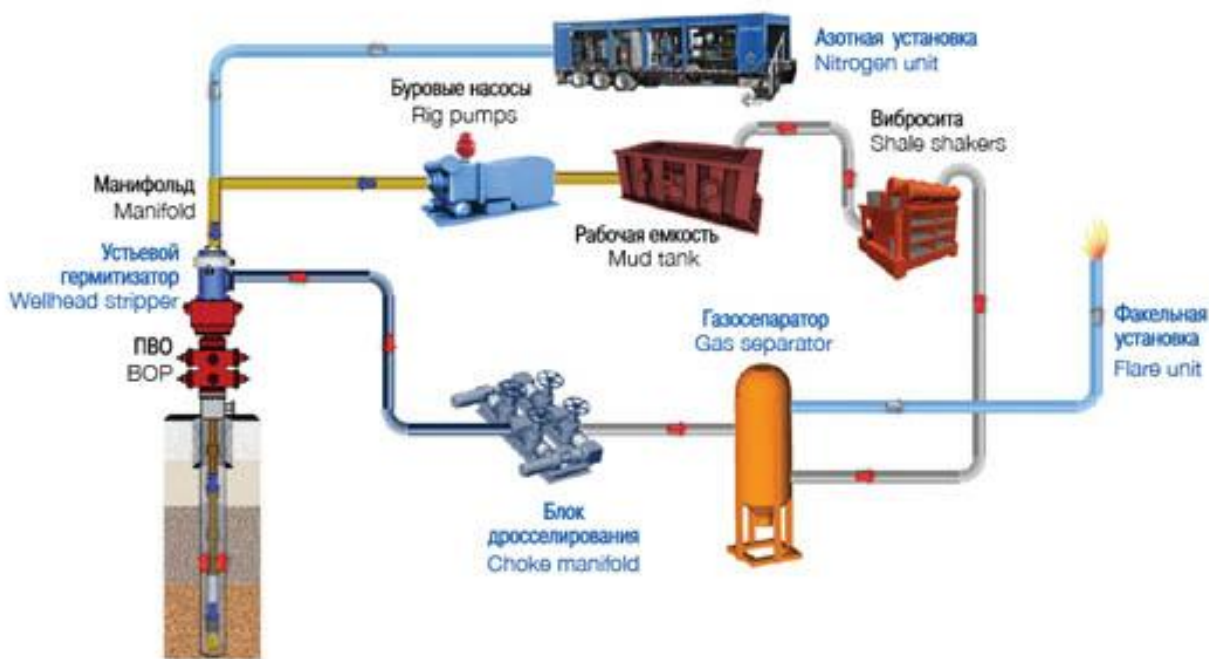
Рисунок 5 - Схема обвязки скважины с системой БРД [5]
